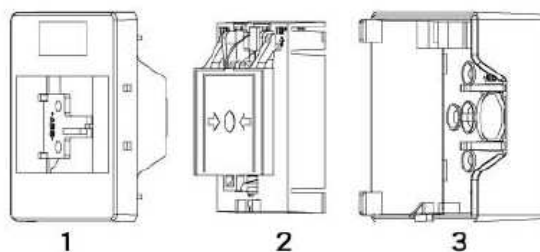
(1/3 – caixa; 2- componente eletrônico) Fig. 4.5.2. Vista explodida
