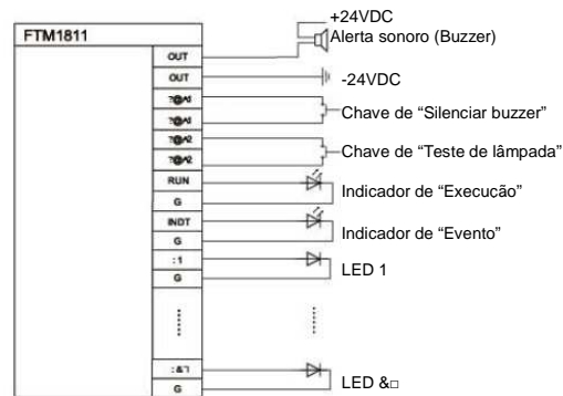
Fig.4.8.4 Diagrama de conexão 1
