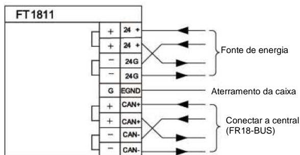
Fig.4.7.2 Diagrama de conexão
