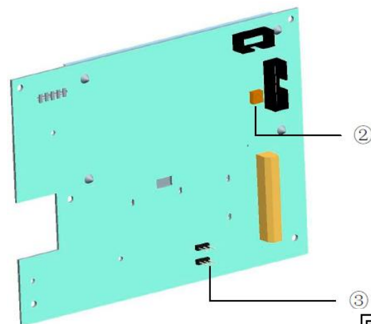
Fig. 3 Vista traseira do Painel PCB
